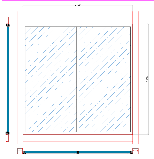
MÓDULO TIPO - SISTEMA CARPINTERÍA AD-HOC 68X54 mm
