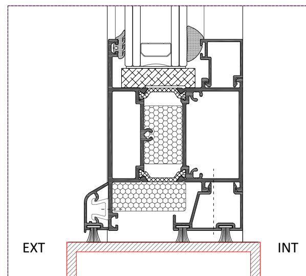
Detalle Sección ESCALA 1:1
