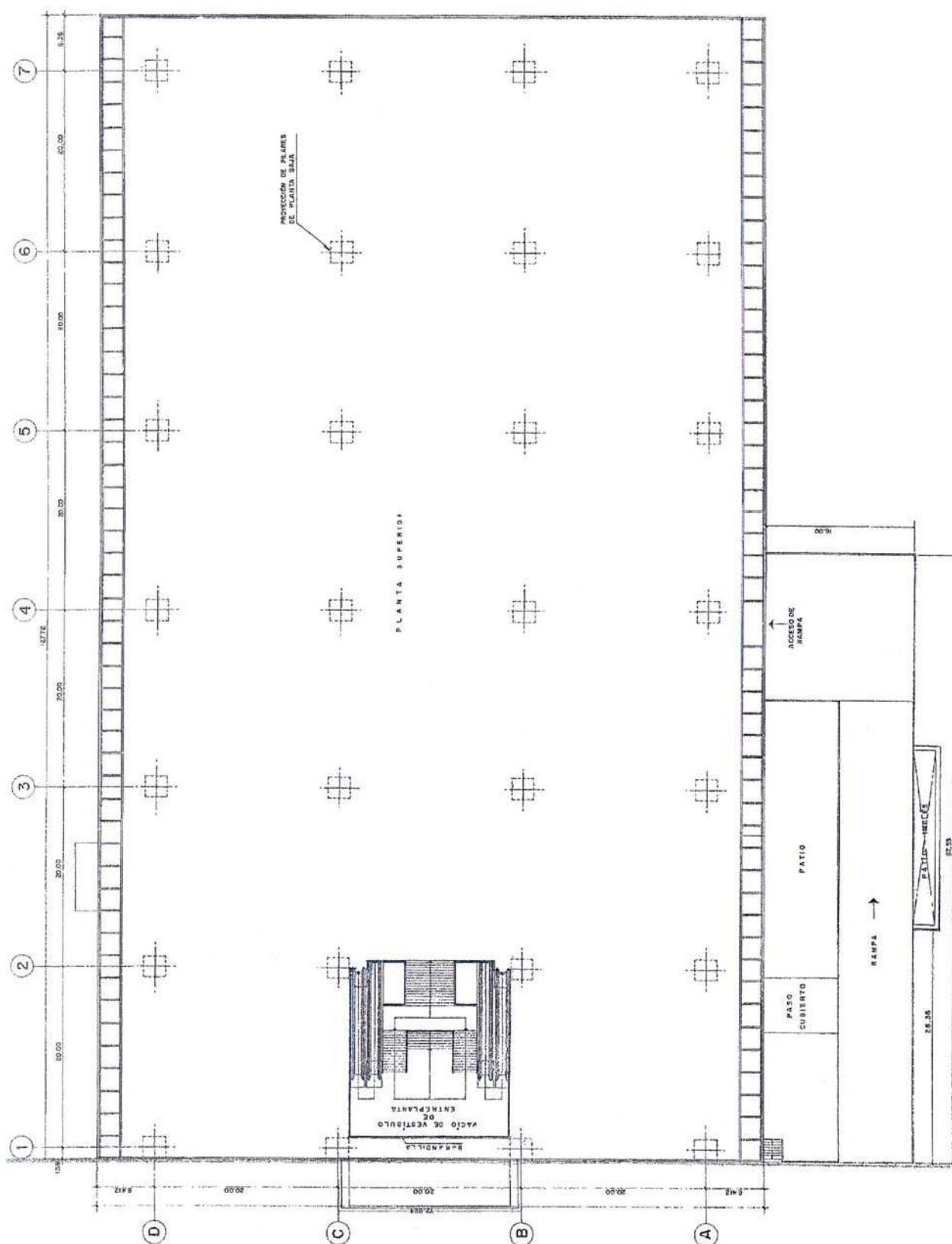
Planta Alta – Proyecto Construido 1965
