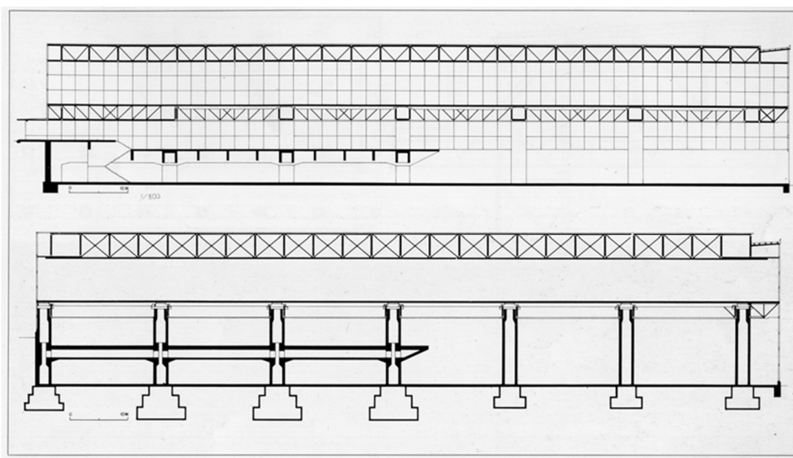
secciones longitudinales
