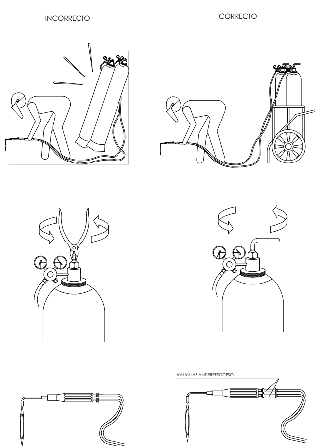
DETALLE 7.1. INSTRUCCIONES GRÁFICAS BOLSAQUERA
