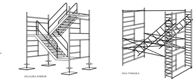
ANDAMIOS METÁLICOS TUBULARES
