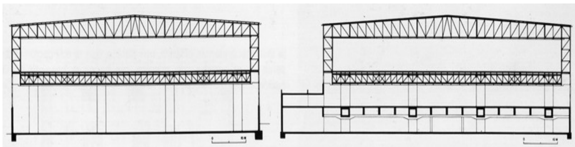
secciones transversales
