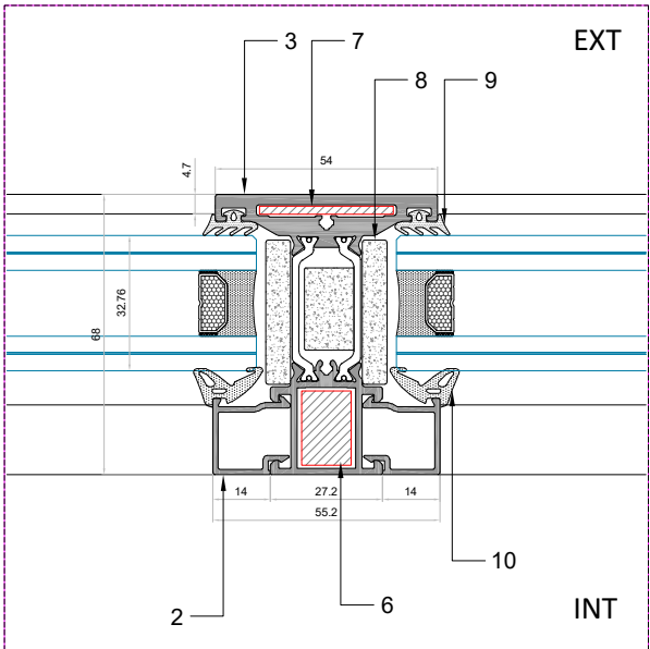
Travesaño 3 - lx: 96,51 cm4 / Wx: 25,39 cm3
