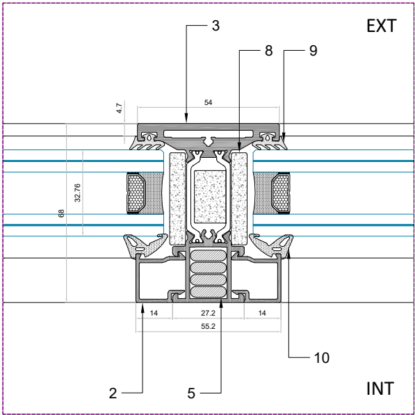
Travesaño 1 - lx: 50,93 cm4 / Wx: 14,22 cm3
