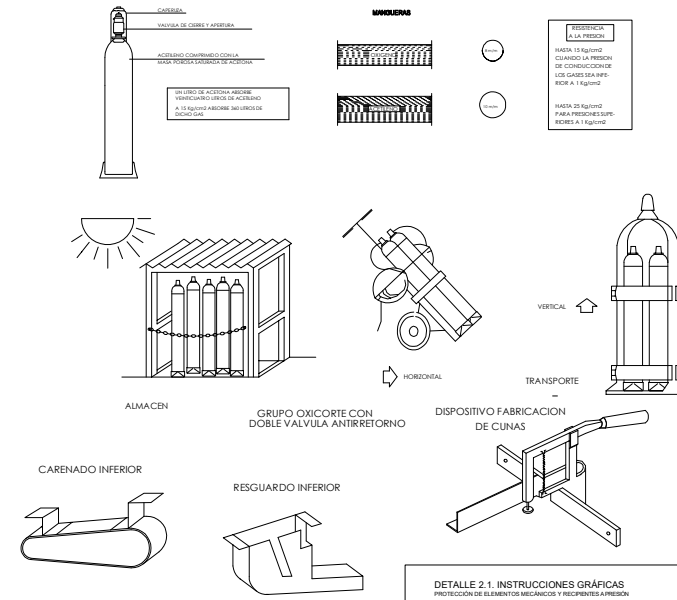
DETALLE 2.1. INSTRUCCIONES GRÁFICAS PROTECCION DE ELEMENTOS MECANICOS Y RECEPTORES A PRESION
