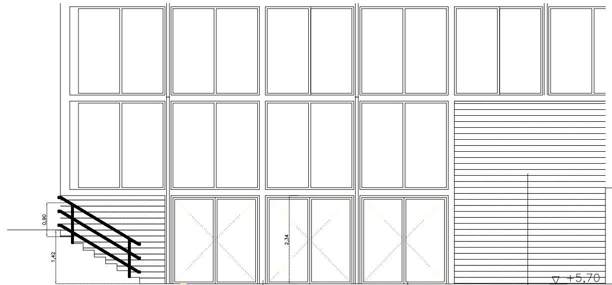
alzado sur
