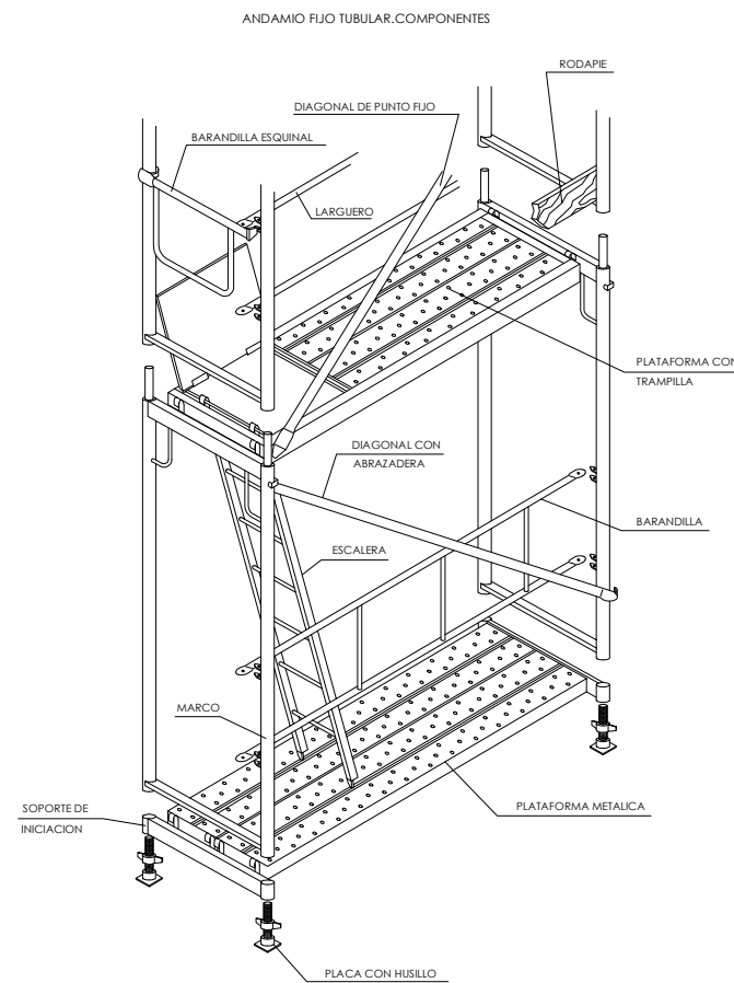
DETALLE 8.1. PLATAFORMAS DE TRABAJO ANDAMIOS TIPO FUSO Y MÓVILES
