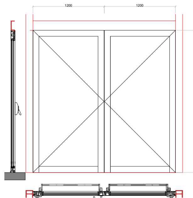
MÓDULO TIPO - SISTEMA CARPINTERÍA PUERTAS TIPO ESCALA 1:20
