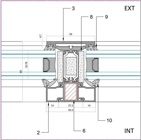
Travesaño 2 - lx: 77,82 cm4 / Wx: 21,73 cm3
