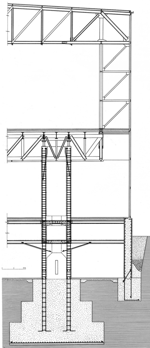
sección constructiva
