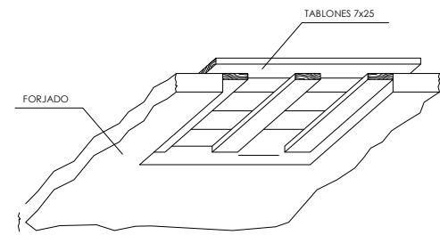
PROTECCION CON TABLEROS
