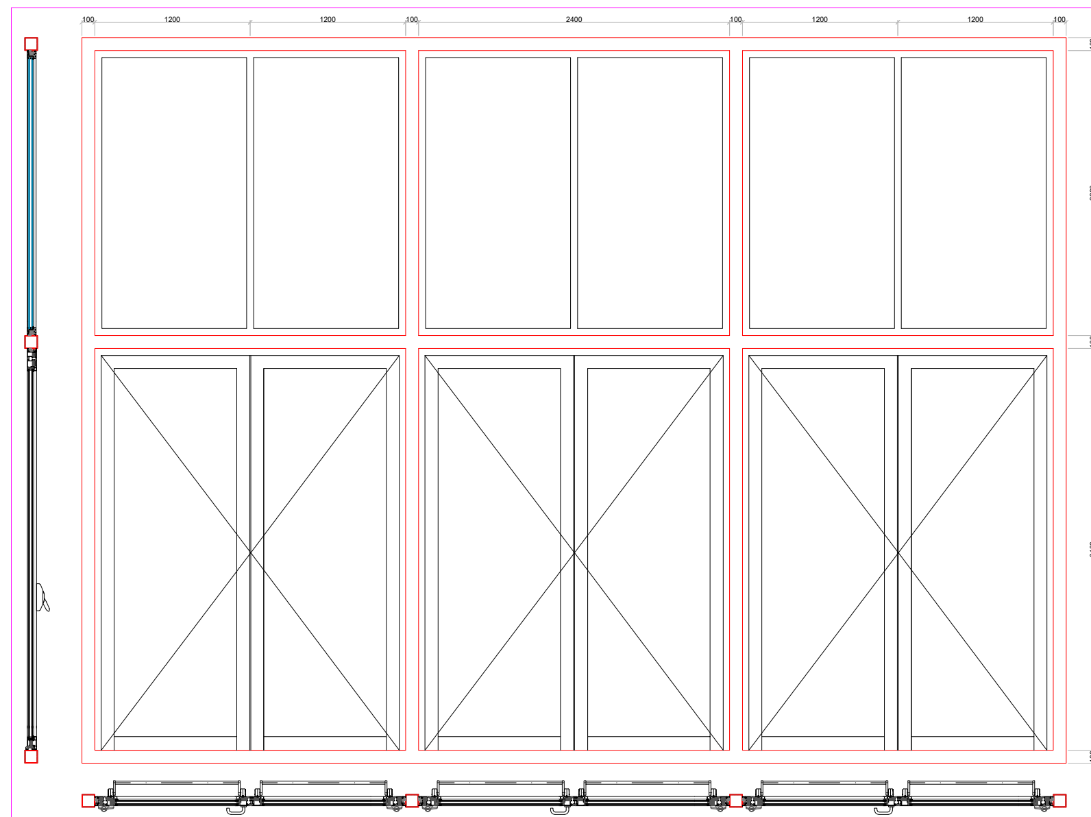
MÓDULO TIPO - SISTEMA CARPINTERÍA PORTONES TIPO ESCALA 1:20
