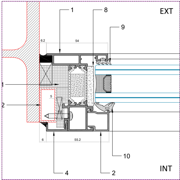
Detalle Planta
