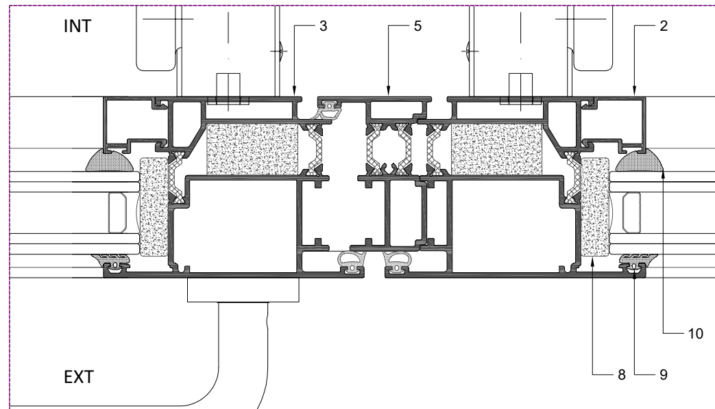
Detalle Planta ESCALA 1:1
