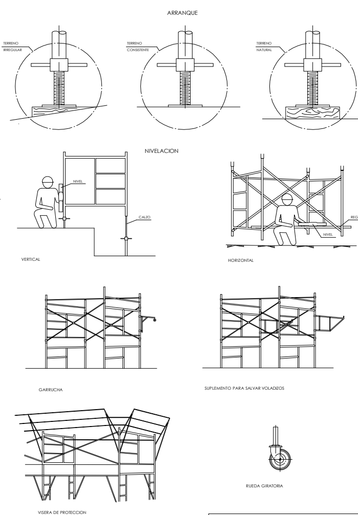
DETALLE 10.2. PLATAFORMAS DE TRABAJO DETALLES DE ELEMENTOS DE ANDAMIOS
