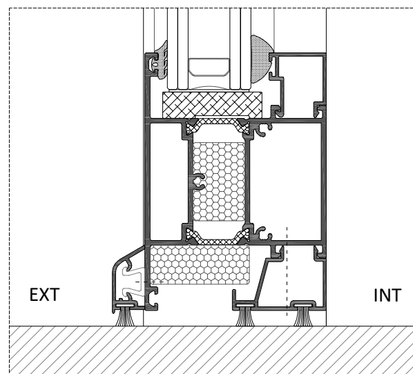
Detalle Sección ESCALA 1:1
