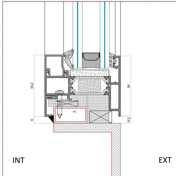
Detalle Sección
