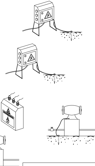
DETALLE 6. INSTRUCCIONES GRÁFICAS PUESTA A TIERRA DE CUADROS Y MÁQUINAS
