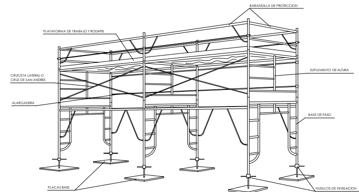
ANDAMIOS METÁLICOS TUBULARES
